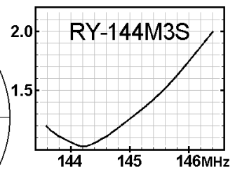
VSWR 特性
